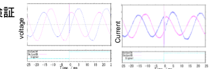
位相差がある電力の切り替え時波形
