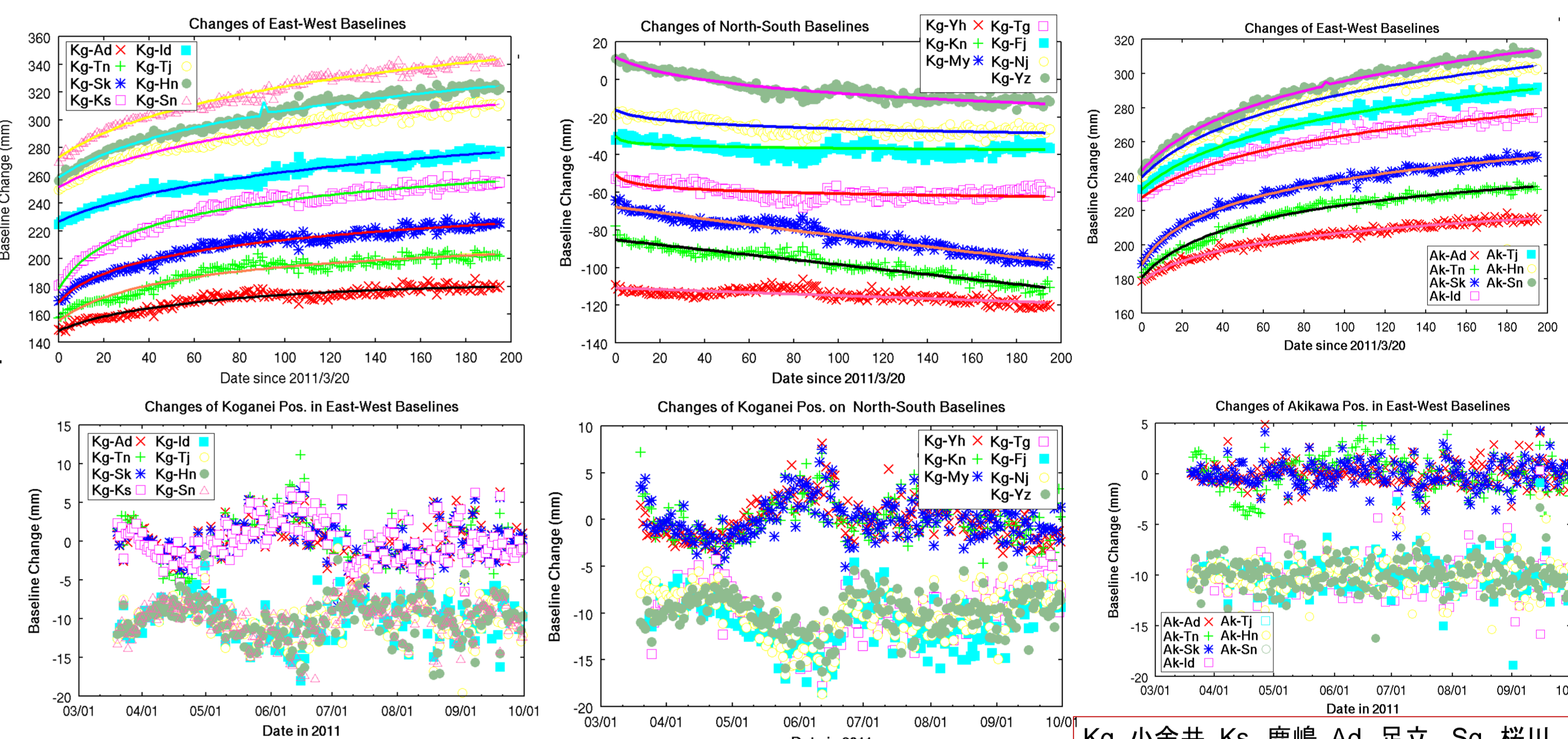
図6 左から小金井を含む東西基線、小金井を含む南北基線、秋川を含む東西基線。上段は基線長の変化であり、下段は滑らかな変動を差し引いた残差。小金井を含む基線にのみ変動がある。小金井局を境に東西で極性が逆転しており、原因が小金井局にあることがわかる。
