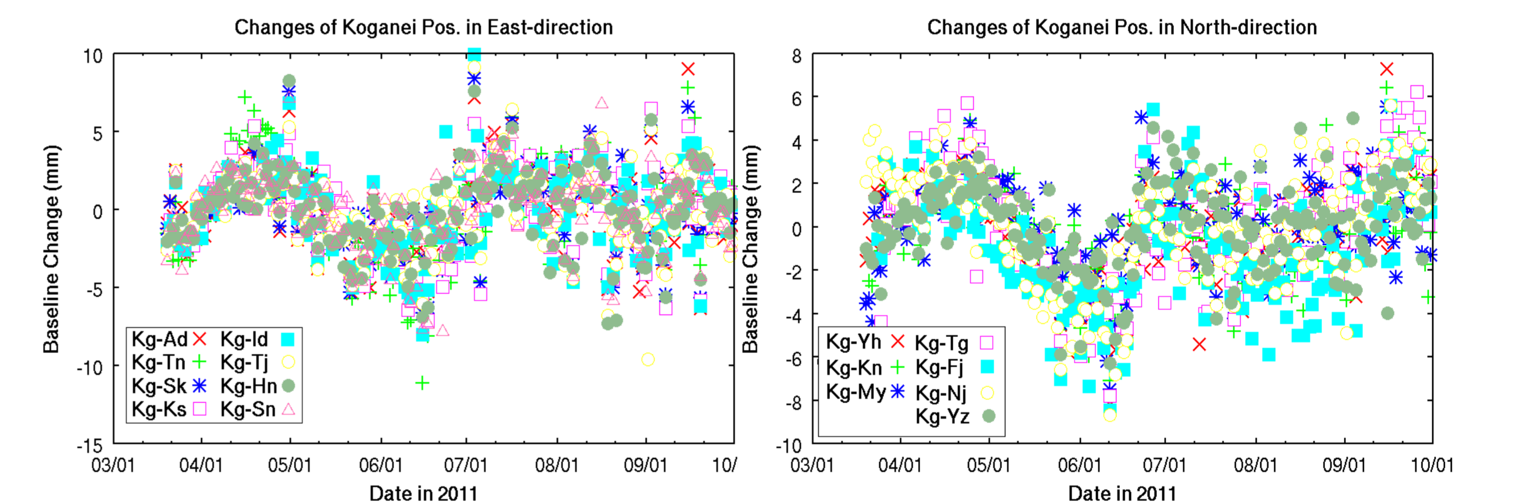
図7 小金井局より東北の基線変化の符号を逆転すると、西(南)側の基線変化と一致する。これが、小金井局の東北の方向の変位であり、振幅5mm周期約3か月で変化している。
