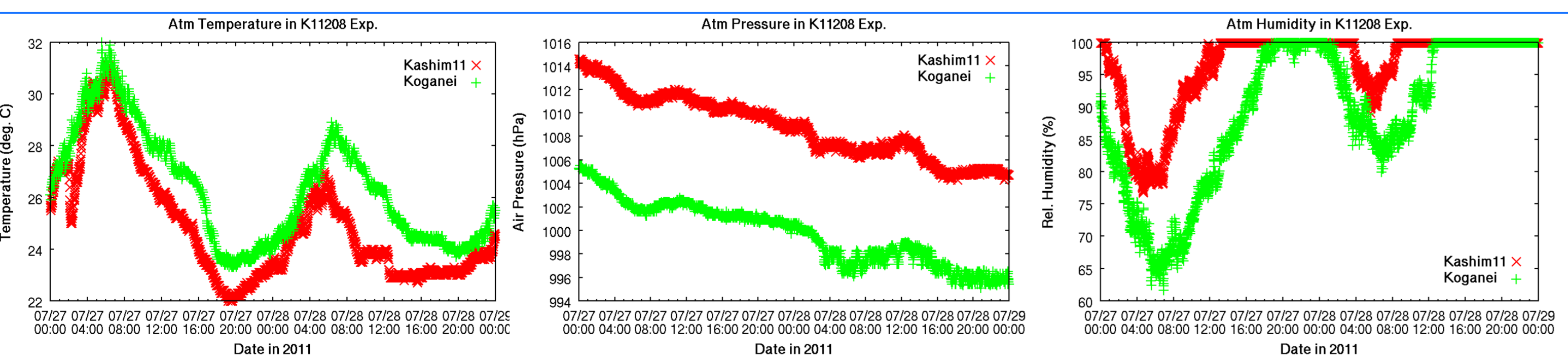
図3 7月27日の気象データ(気温、気圧、湿度)。
