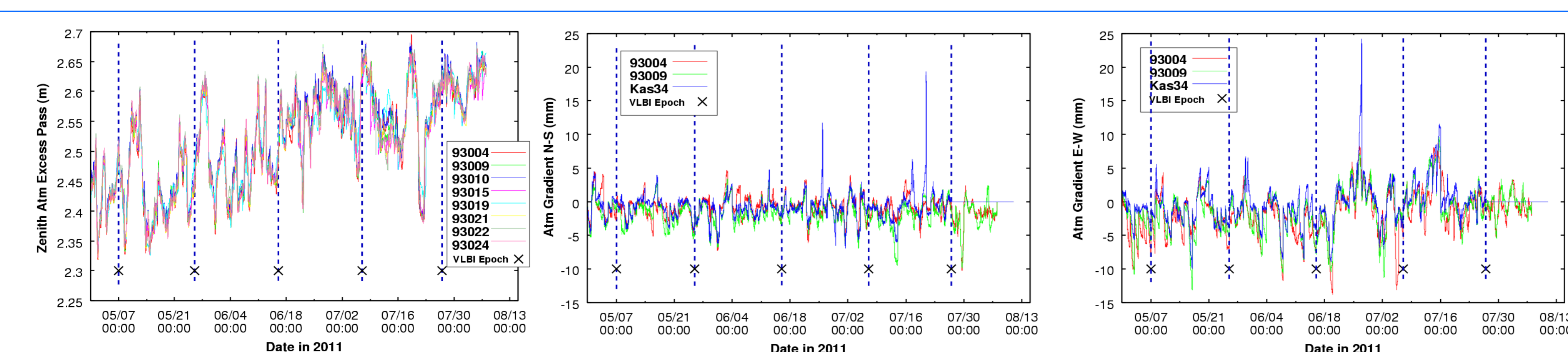
図4 GPSのPPP解析によって得られた大気天頂ExcessPassと大気勾配の推定値。VLBI観測日時に縦線を入れている。VLBI観測の日時で特に目立った大気遅延量・変化は観測されていない。
