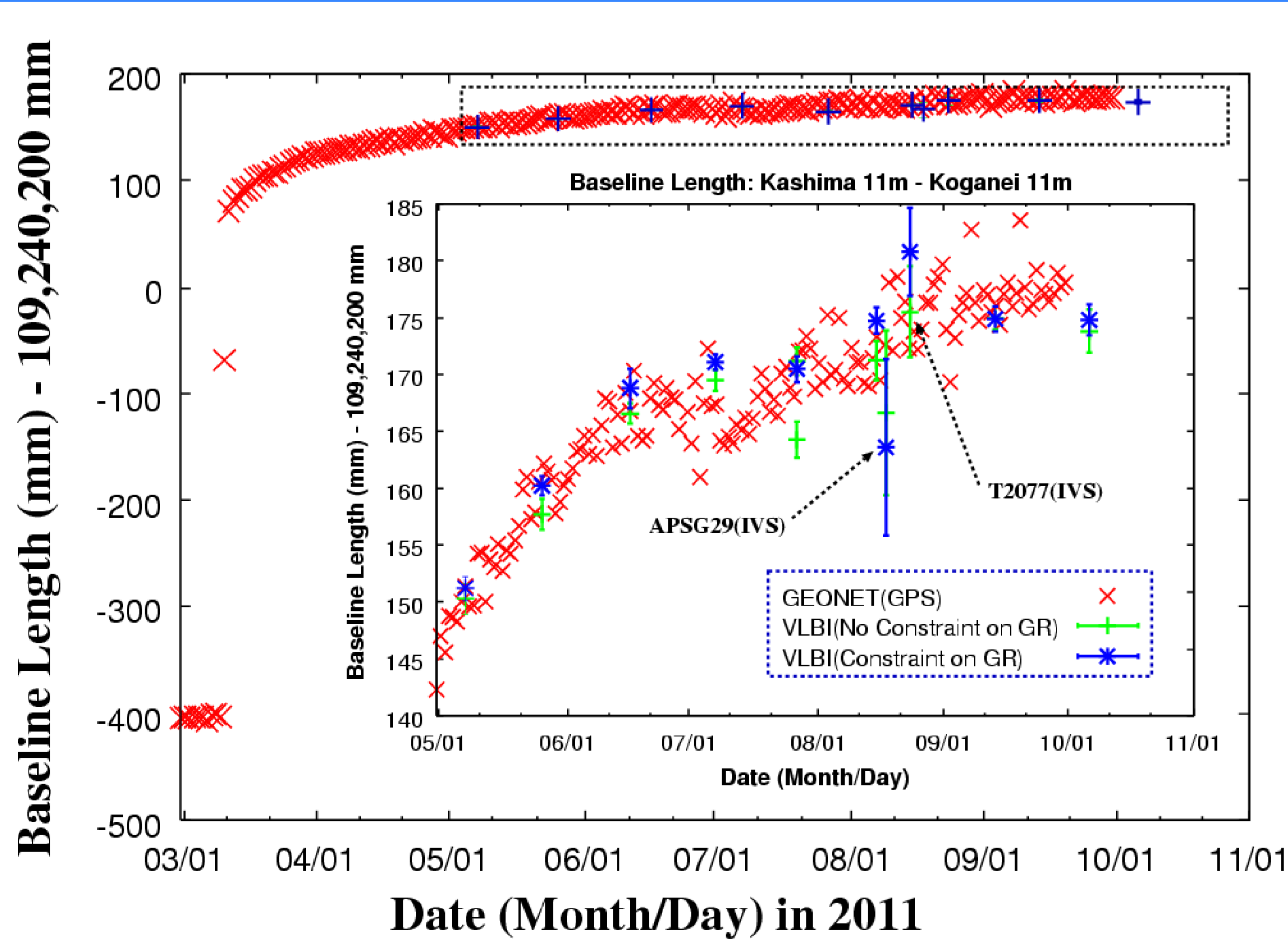
図2 鹿島一小金井基線のVLBI解析結果とGEONETの鹿島一小金井基線。大気勾配の拘束条件なしで推定を行った場合には基線長推定値に影響を与えて、見かけ上基線が短縮したように見える結果が得られることがある。
