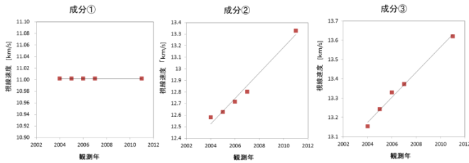
図 5.長期で見た Mon R2 の視線速度の変化
