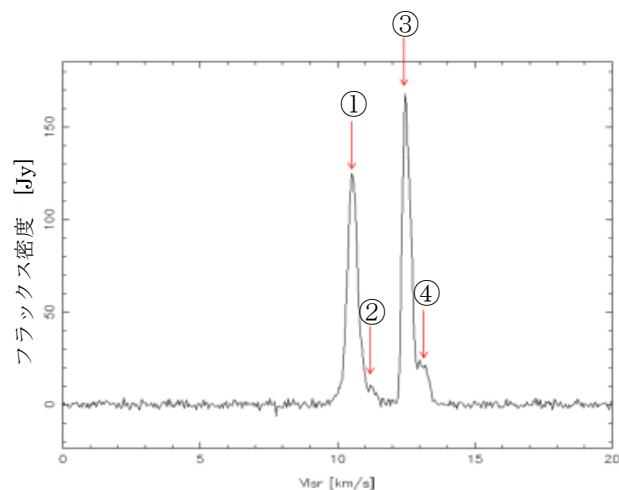
図 3. Mon R2 の通算日 279 におけるスペクトル
