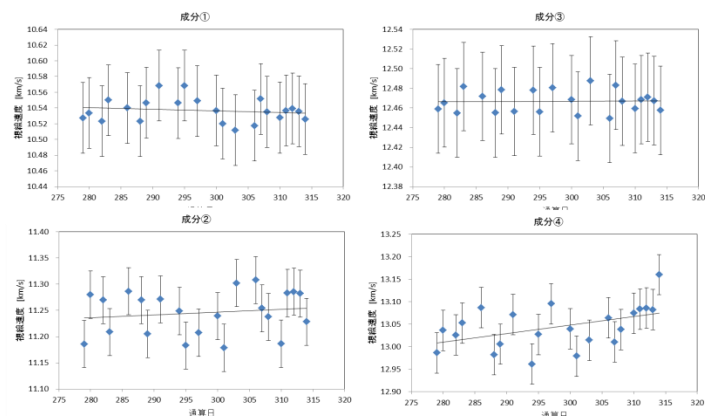
図 4. 各成分における視線速度の変動
