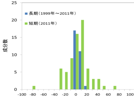
図 6.長期・短期での視線速度の変化率
