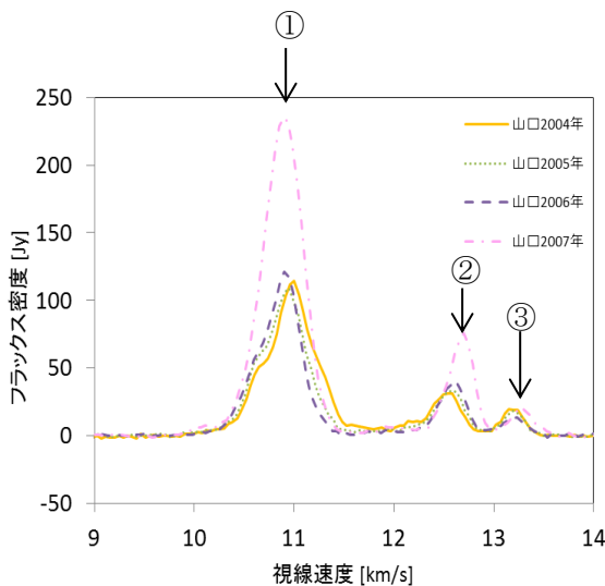
図 7 .Mon R2 のスペクトル
