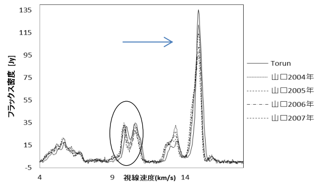
図 1. 14.09 + 0.10 における Torun 及び山口 32m のスペクトル
