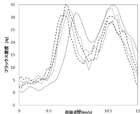
図 2. 図 1 の○で囲った範囲の拡大
