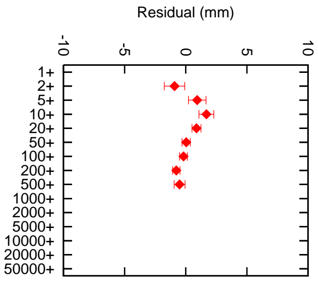
Matera 7941 LAG1+LAG2
