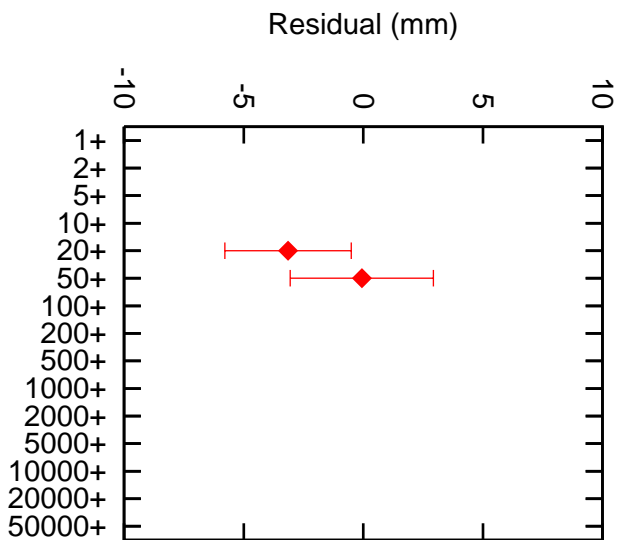
Maidanak 1864 STRL+STEL
