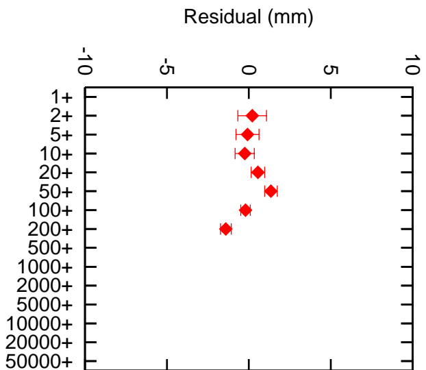
Greenbelt 7105 LAG1+LAG2
