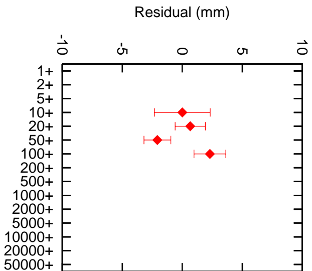
Maidanak 1864 LAG1+LAG2
