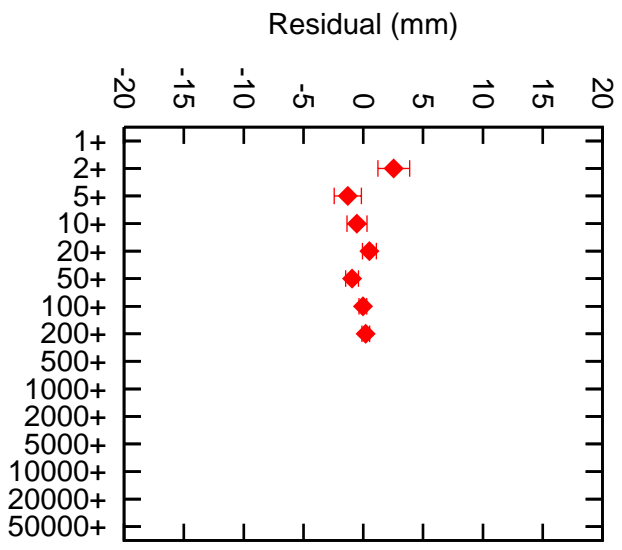
Matera 7941 AJI
