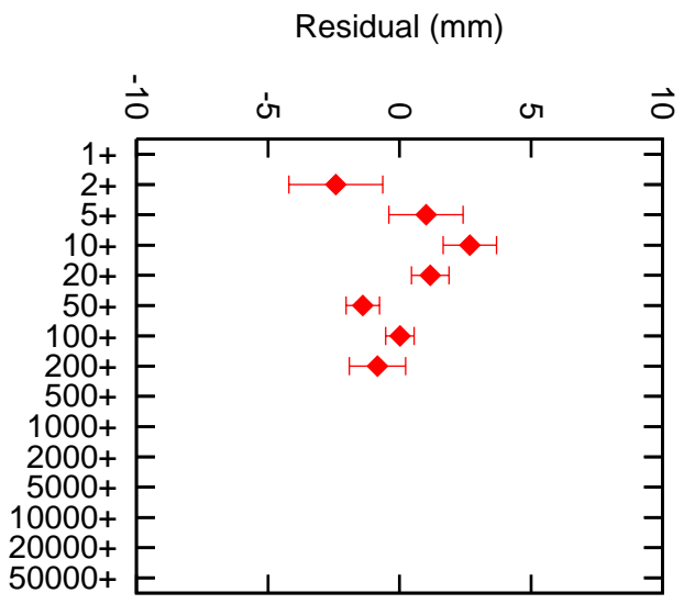
Matera 7941 STRL+STEL
