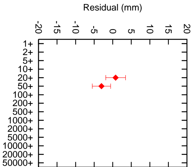
Maidanak 1864 AJI
