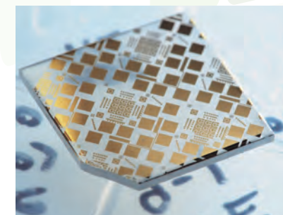
酸化ガリウムトランジスタ、ダイオードを作製したチップ
