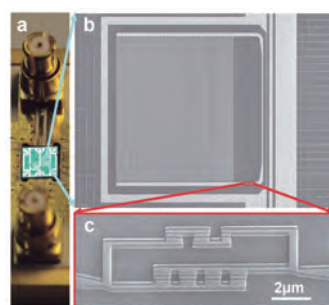
実際に用いた試料と回路素子 a. 試料ホルダーに装填された測定チップ b. 深強結合 qubit (赤枠箇所)-LC調和振動子回路、アルミニウム製 c. 超伝導 flux-qubit
