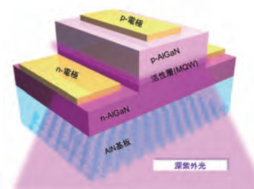
深紫外LEDデバイス構造
