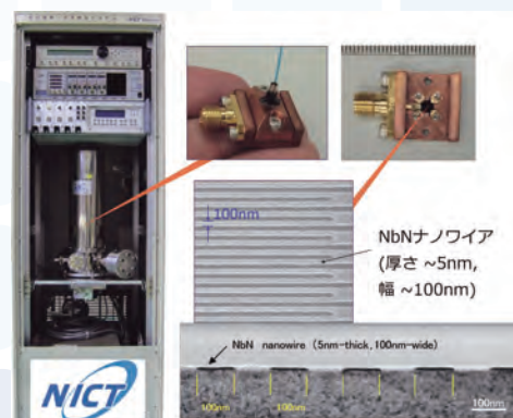
超伝導単一光子検出器システム
