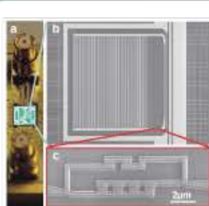
実際に用いた試料と回路素子 a. 試料ホルダーに装着された測定チップ b. 深強結合 qubit (赤枠箇所) - LC 共振器と振動子回路、アルミニウム製 c. 超伝導 flux-qubit
