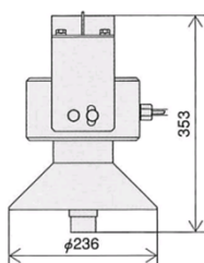
■ 送受波器 (TUS-200S) 外形図
