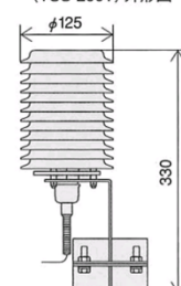
■ 温度計 (TUS-200T) 外形図
