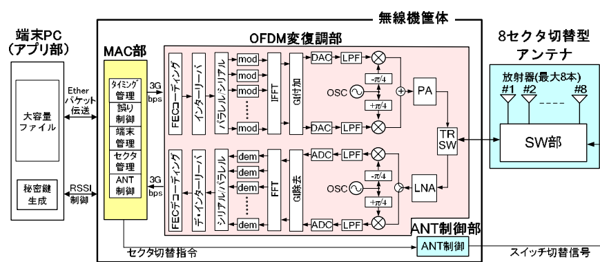
無線機の構成ならびに要素技術
