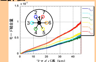
図 中心コアへ光パルスを励起した際の周辺コアへのモード結合量
