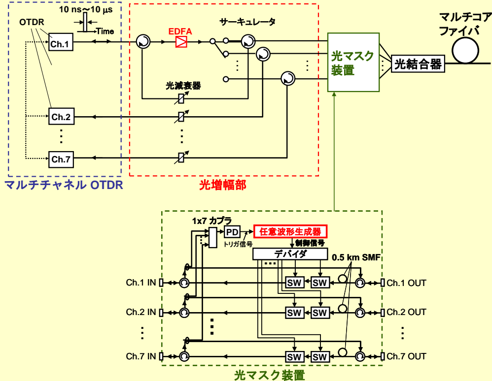
図 改良したOTDRを用いたマルチコアファイバの長手特性評価系の構成
