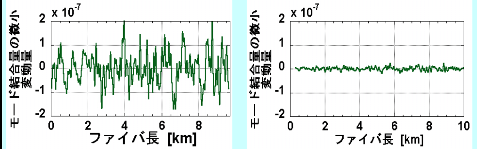
(a)ファイバ構造揺らぎ=大
