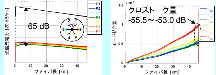
図 中心コアに光パルスを励起した際の各コアからのレイリー散乱光電力(左)および周辺コアへのモード結合量(右)
