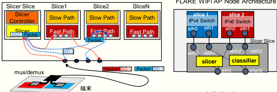
FLAREを使用したWiFiアクセスポイント仮想化
