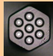
六角形マルチコアファイバ
