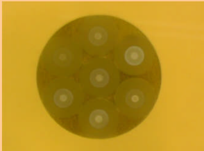
フェルール孔構造の変更による加工作業性の向上
