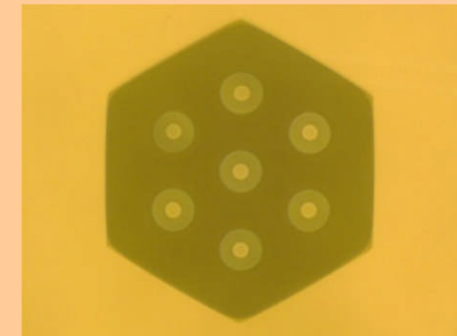
端末加工後フェルール端面
