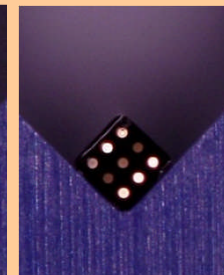
矩形9コアマルチコアファイバ 90° V溝
