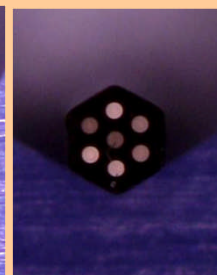
六角形マルチコアファイバ 120° V溝
