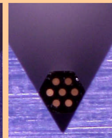
六角形マルチコアファイバ 60° V溝
