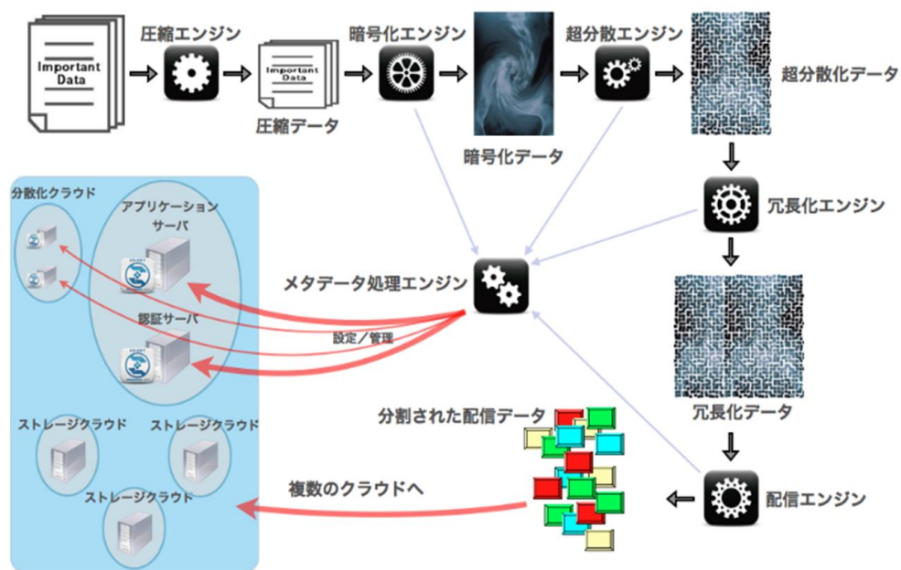
図 2 ディザスタリカバリシステム
