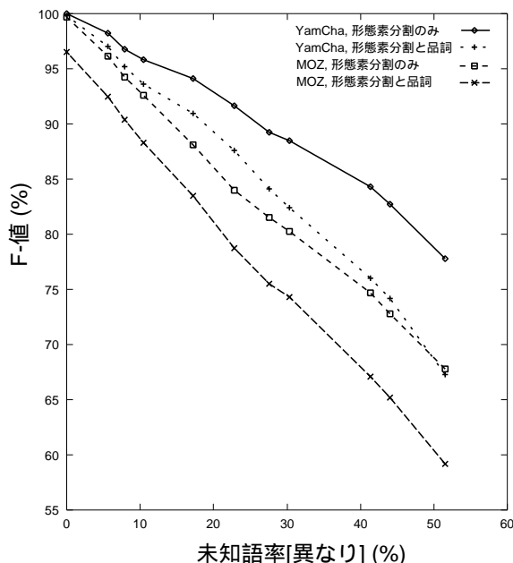
図 2 未知語率 [異なり] と解析精度
