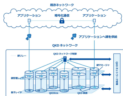
QKDネットワークの概略
