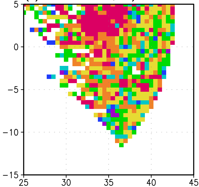
(f) Dif. MAG( \vec{u}, \vec{v} ): CE-SO
