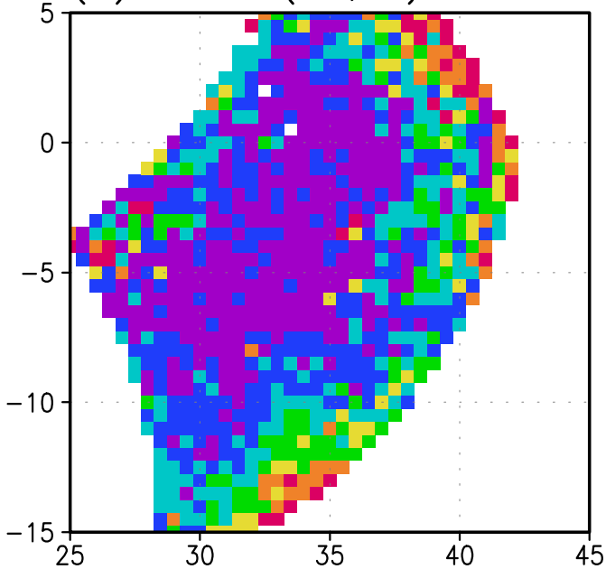
(d) Dif. MAG( \vec{u}, \vec{v} ): NO-CE
