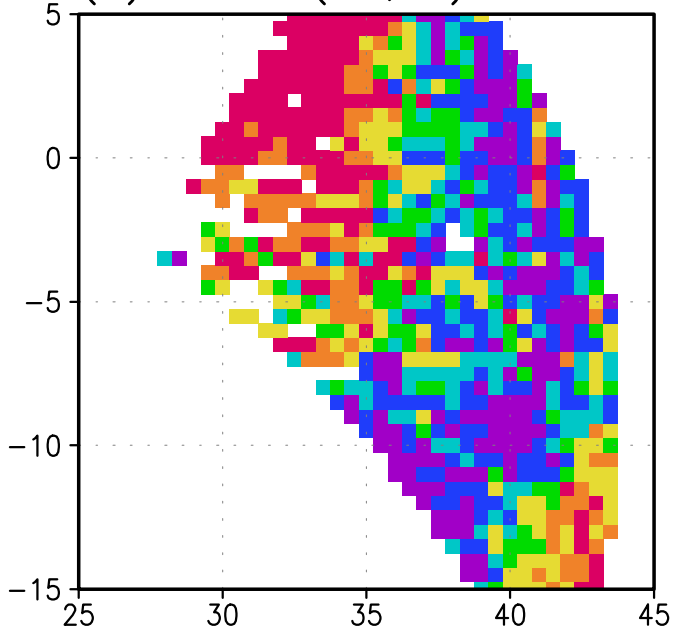
(e) Dif. MAG( \vec{u}, \vec{v} ): NO-SO
