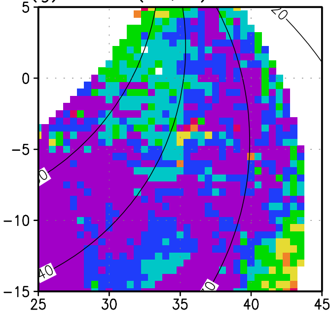
(g) Dif.MAG(du,dv): NO-COMP
