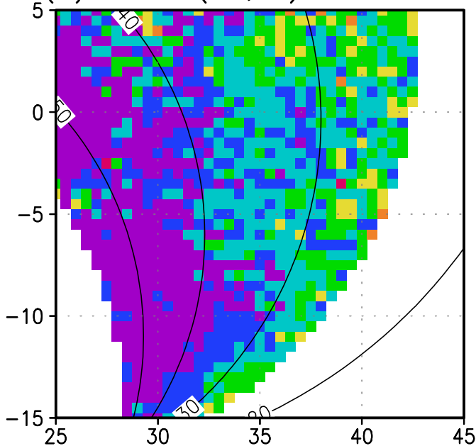
(h) Dif.MAG(du,dv): CE-COMP
