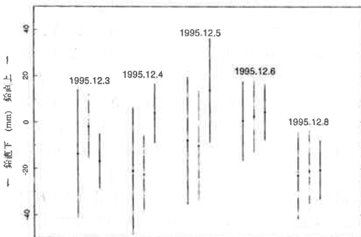
第6図 自動解析とマニュアル解析，従来のシステムによる解析結果の比較。小金井局推定位置の鉛直成分。それぞれの実験について、左から自動解析，マニュアル解析，従来のシステムによる解析の結果を示す。原点は ITRF 93 座標系における小金井局の位置にとった。
