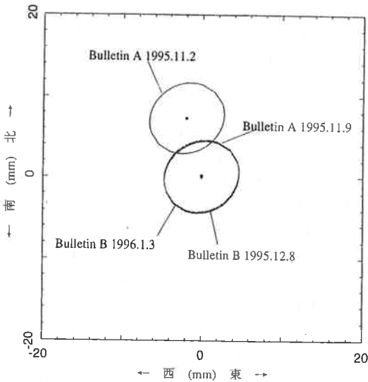
第8図 異なる IERS Bulletin の地球回転パラメタを使用したときの解析結果の比較。水平面内における小金井局の位置。原点は、1996年1月3日に発行された Bulletin B の値で解析した結果をとった。
