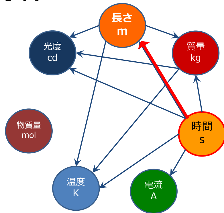
SI国際単位の依存関係(2019~)
