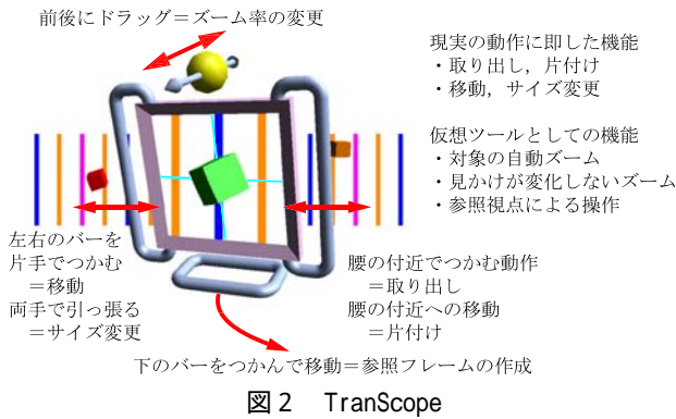
図 2 TranScope
